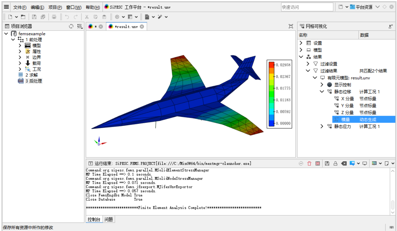
图 5.8 位移云图
